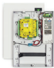
Net2 plus 1 deur deurcontroller - 12V 2A voeding, kunststof behuizing
